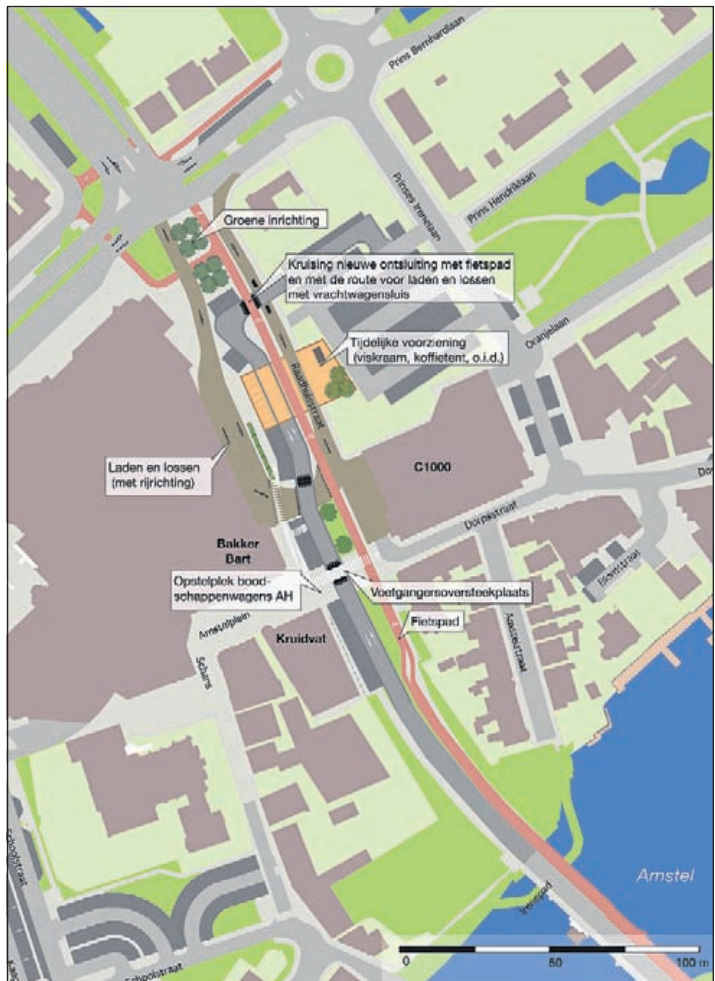
Overzichtsplan van de tijdelijke herinrichting van de N196 in het centrum van Uithoorn.
