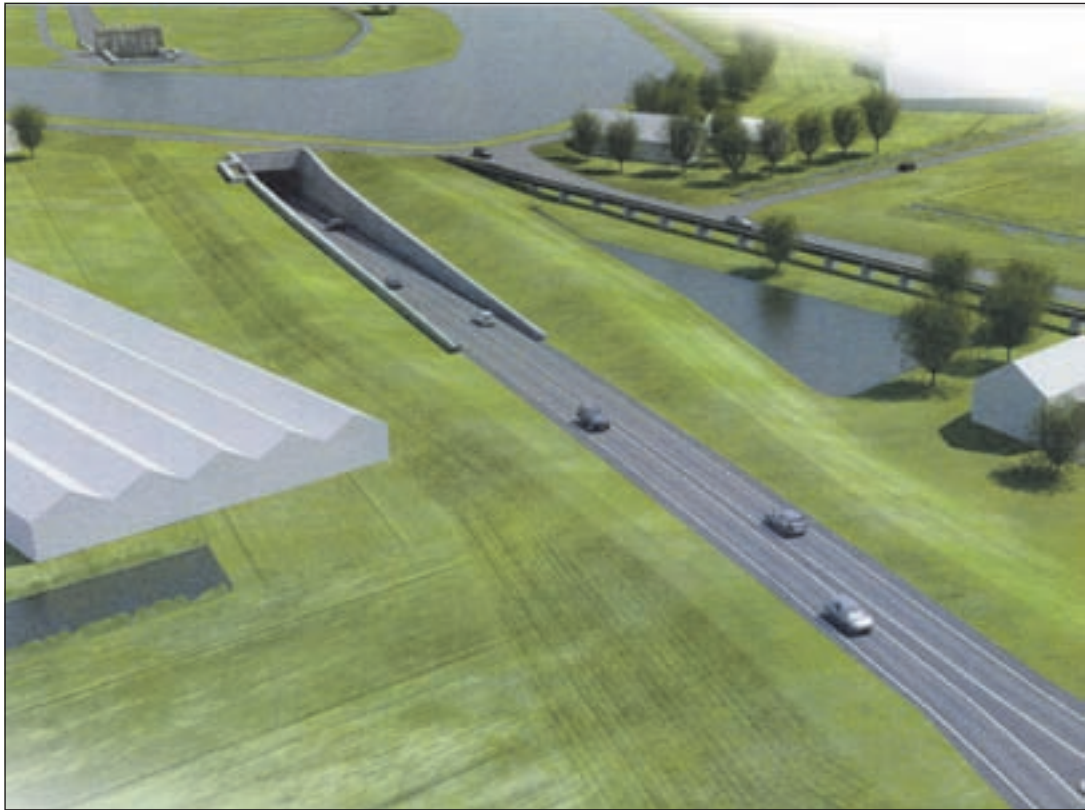
Impressie van de N201, omlegging Amstelhoek met aquaduct. Rechtsboven de Hollandse Dijk met de bestaande afwateringsgoot
