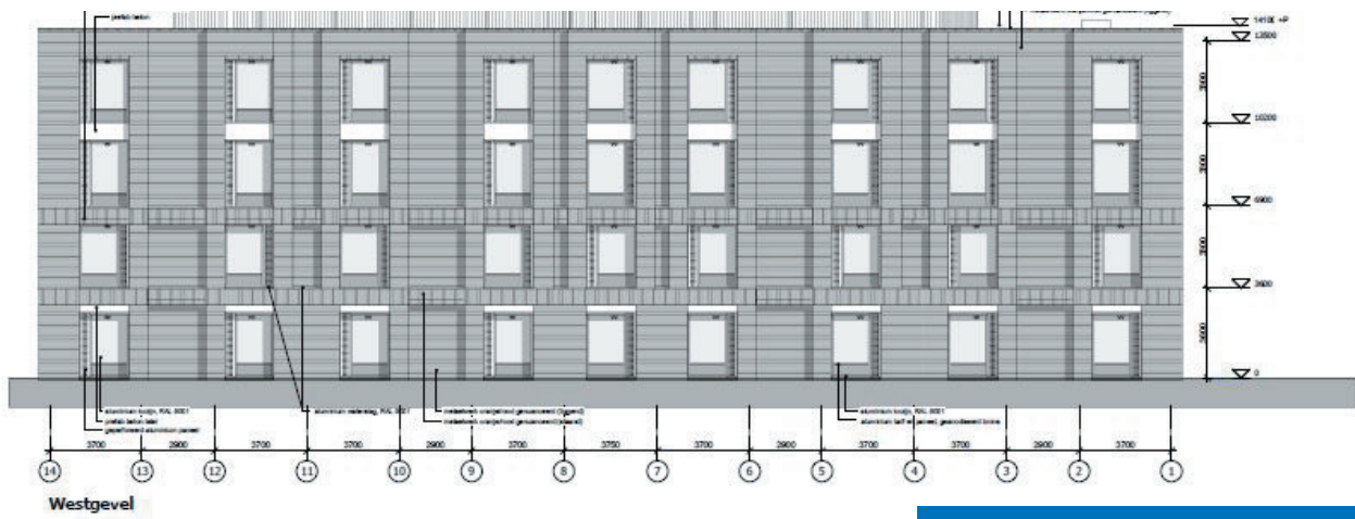
AANZICHTEN ZUID- EN WESTGEVEL
