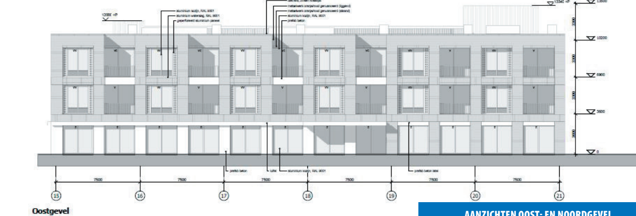
AANZICHTEN OOST- EN NOORDGEVEL
