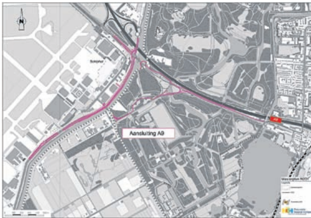
Overzicht van de nieuwe aansluitingen vanaf de Fokkerweg op de A9
