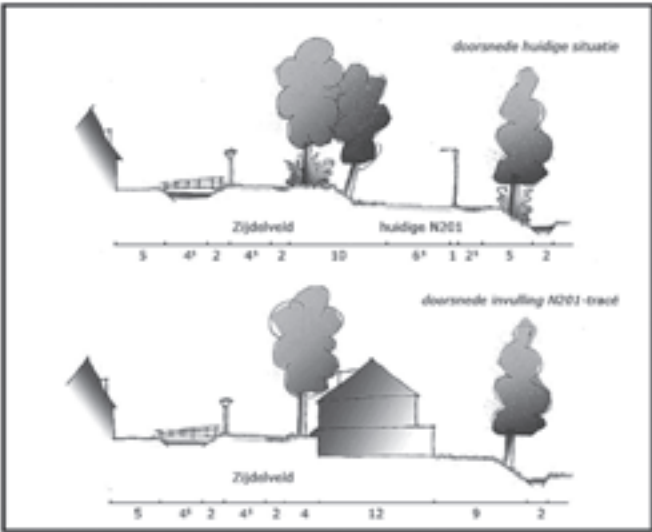
Figuur 9: Dwaarsdoorsneden Zijdelveld en huidige N201-tracé
