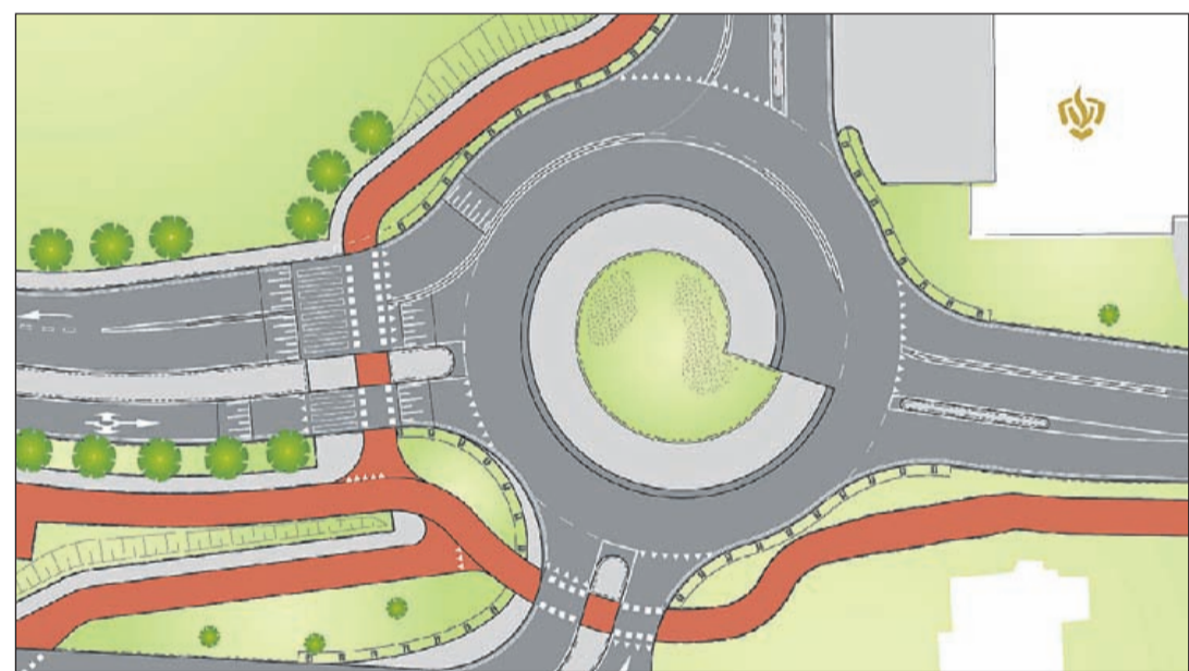
Impressie van de rotonde hoe deze er op 18 september uit ziet. Bovenaan de Industrieweg met er naast de Brandweerkazerne; links en rechts de aansluiting op de Rondweg en onderaan op de Stationsweg (ref. gemeente DRV)
