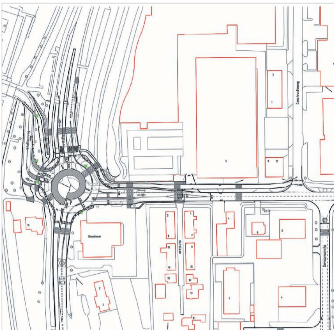
Inpassing rotonde in de verkeersstructuur. Rechts de Industrieweg, boven De Rondweg richting Dukaton, onder de Rondweg richting Rabobank en links de aansluiting op de Stationsweg (ref. gemeente DRV)
