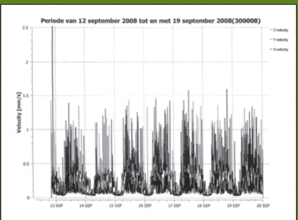
DE TRILLING GRAFIEK UIT HET ONDERZOEK. HET MAXIMALE MAG 1 ZIJN.
