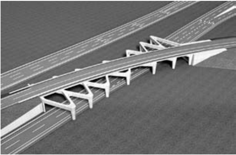
De ‘Pergola’-constructie voor de busbaan (HOV) naar Hoofddorp
