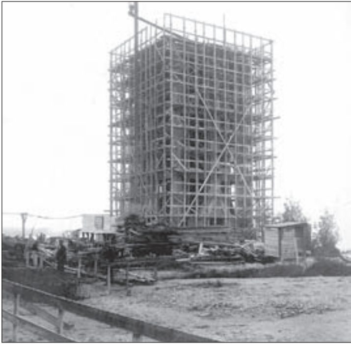
De watertoren van Aalsmeer in aanbouw in 1927 (bron: archief PWN).
